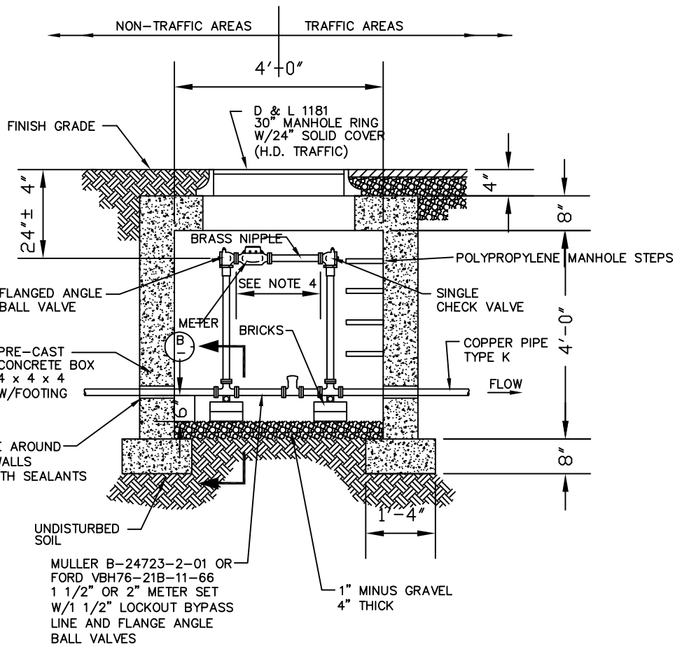
A 1 1/2" & 2" METER VAULT - N.T.S.
