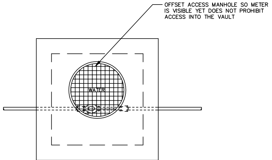
A 1 1/2" & 2" METER VAULT - N.T.S.
